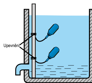
SPÍNÁNÍ VÍCE HLADIN
